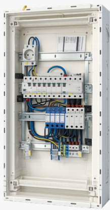
Anschlussfertige 4- und 5-reihige Wohnungsverteiler
