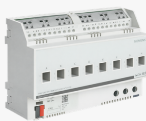
N 534D61 KNX Schaltaktor 12 x AC 230 V, 16/20 AX, C-Last
