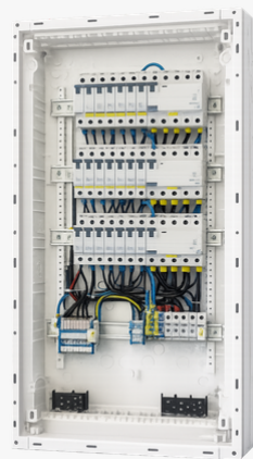
Mit Schraub- oder Steckklemmenanschluss erhältlich
